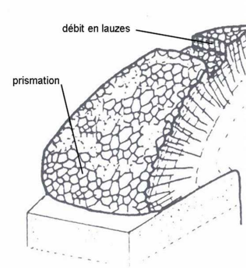
Géométrie des prismes volcaniques sur un dôme phonolitique (A.M. Gonzales, D. Nectoux, H. Bertrand, (2003) - http://planet-terre.ens-lyon.fr/article/orgues-volcaniques.xml )
